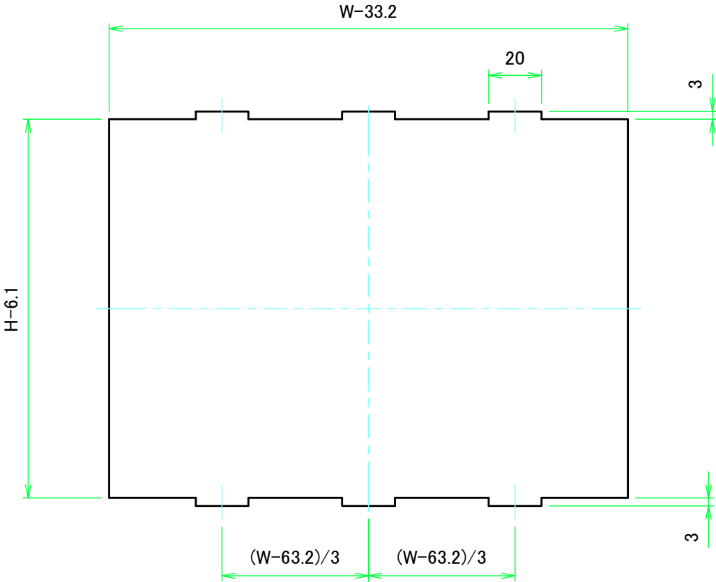
Wパネル1表面 / W Panel 1 Frontside
